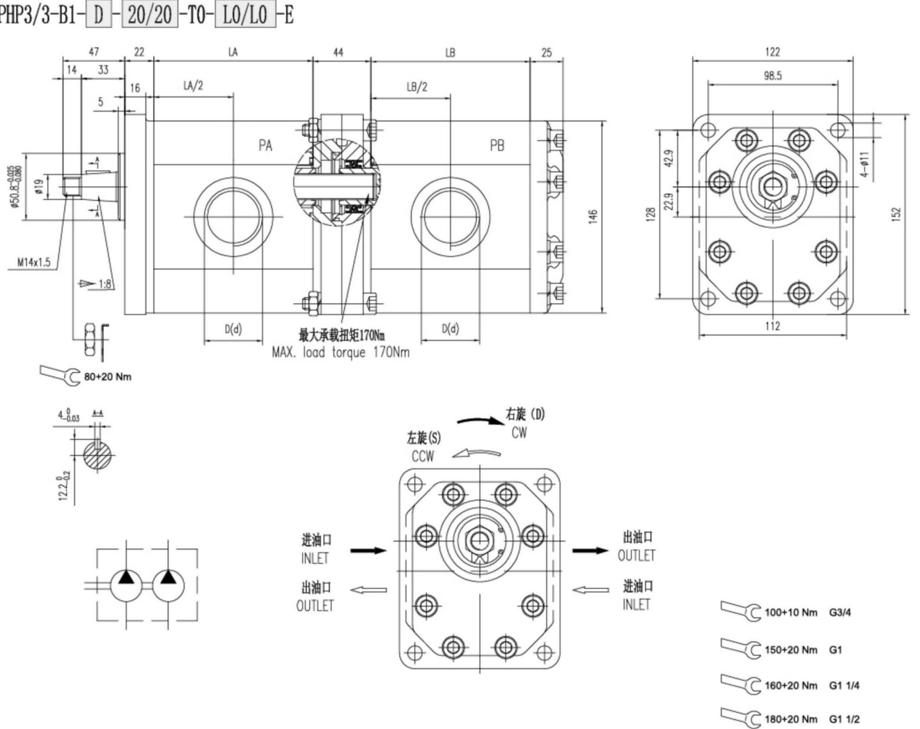
3/3系列标准型产品尺寸/Group 3/3 Standard Product Dimensions
